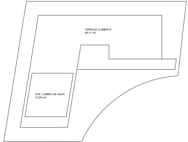
DIAGRAMA SUPERFÍCIES PLANTA CUBIERTA
