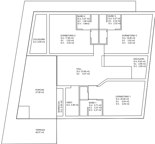
DIAGRAMA SUPERFÍCIES ÚTILES PLANTA BAJA
